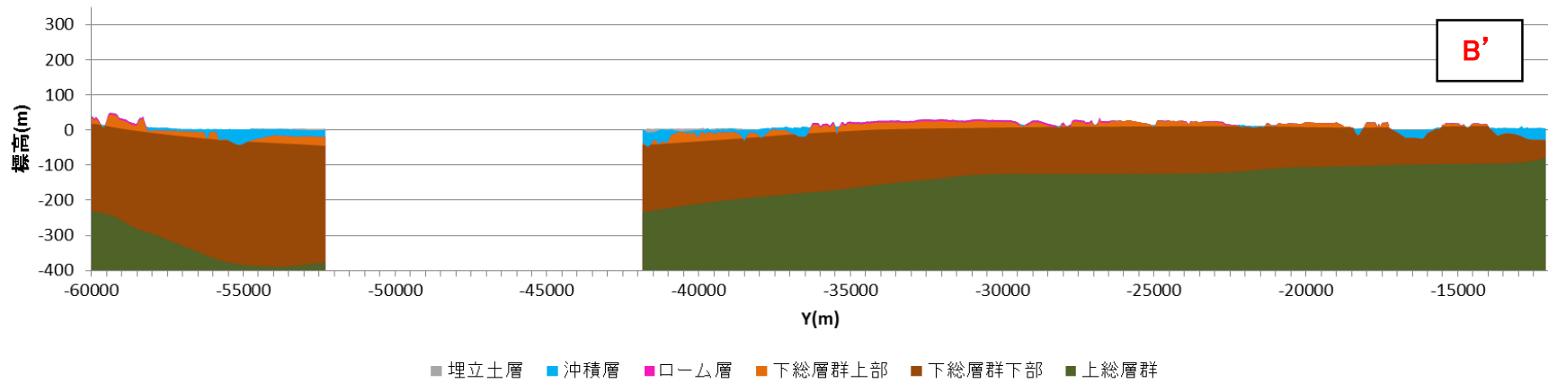
图 3-13 南北方向断面图 (X=20000m · Y=-105000~-12000m) (例)
